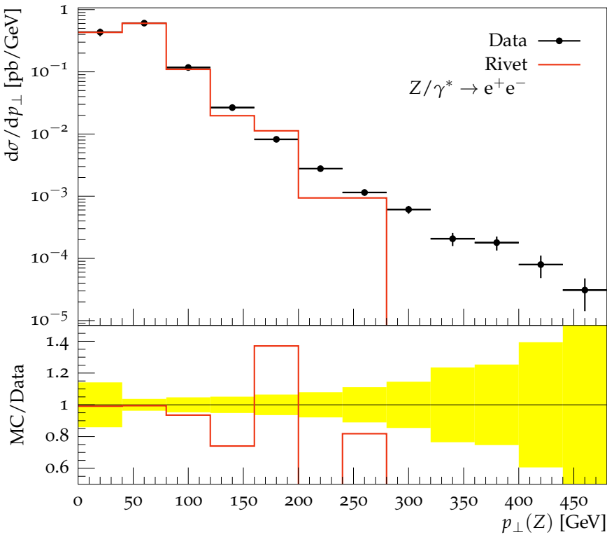
Transverse momentum of Z-boson (Z + 1jet events)
