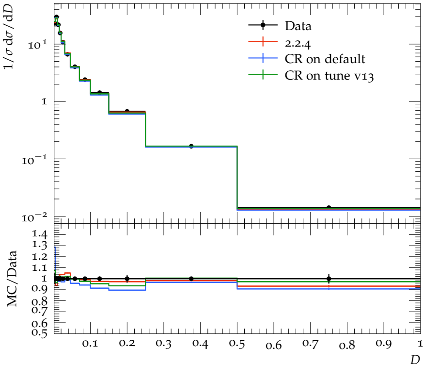
D parameter at 91 GeV
