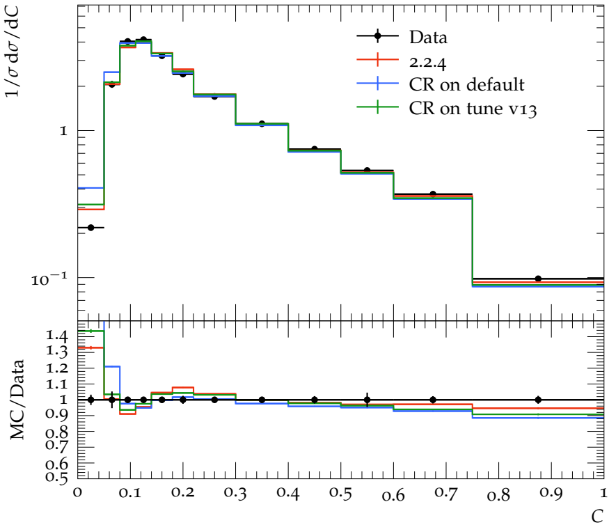
C parameter at 91 GeV
