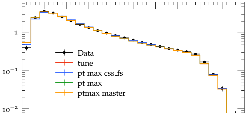
C parameter (charged)
