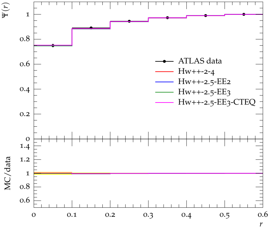
Jet shape \Psi for p_{\perp} \in 310\text{--}400\text{ GeV} , y \in 0.0\text{--}2.8
