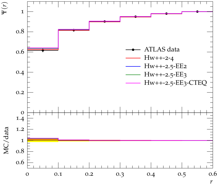
Jet shape \Psi for p_{\perp} \in 110\text{--}160\text{ GeV} , y \in 0.8\text{--}1.2
