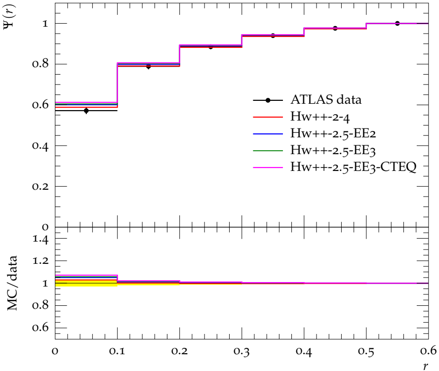
Jet shape \Psi for p_{\perp} \in 80\text{--}110\text{GeV} , y \in 0.0\text{--}2.8
