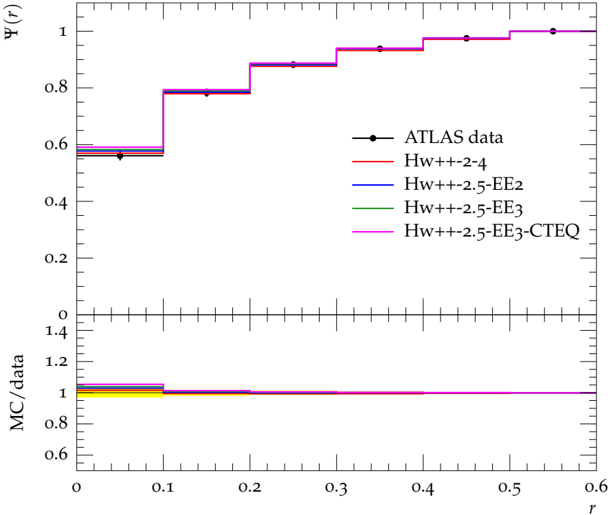
Jet shape \Psi for p_{\perp} \in 80\text{--}110\text{GeV} , y \in 0.3\text{--}0.8
