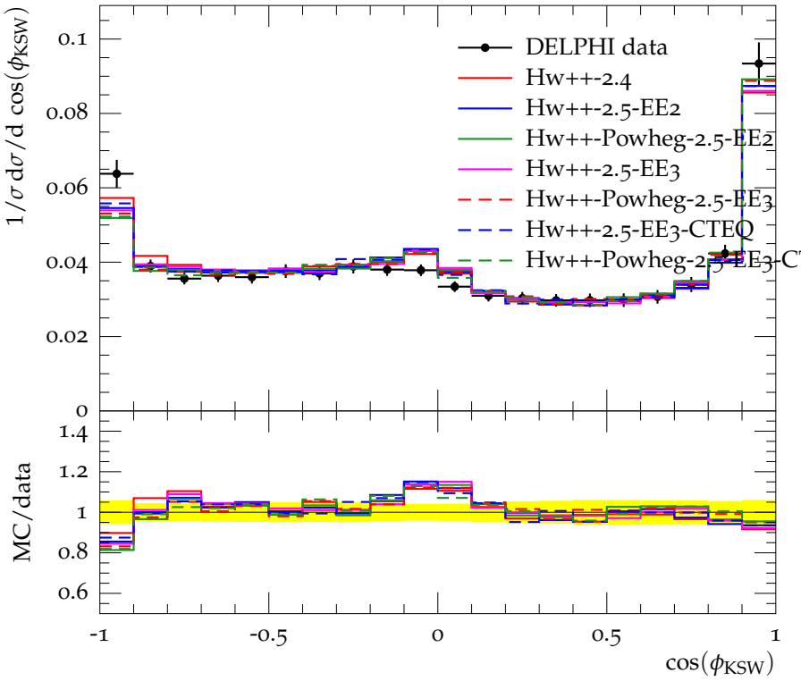
Körner-Schierholz-Willrodt \cos(\phi_{\text{KSW}}) , Durham y_{\text{cut}} = 0.008
